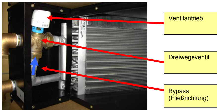
CoolTherm Wärmetauscher Ansicht (von hinten)
